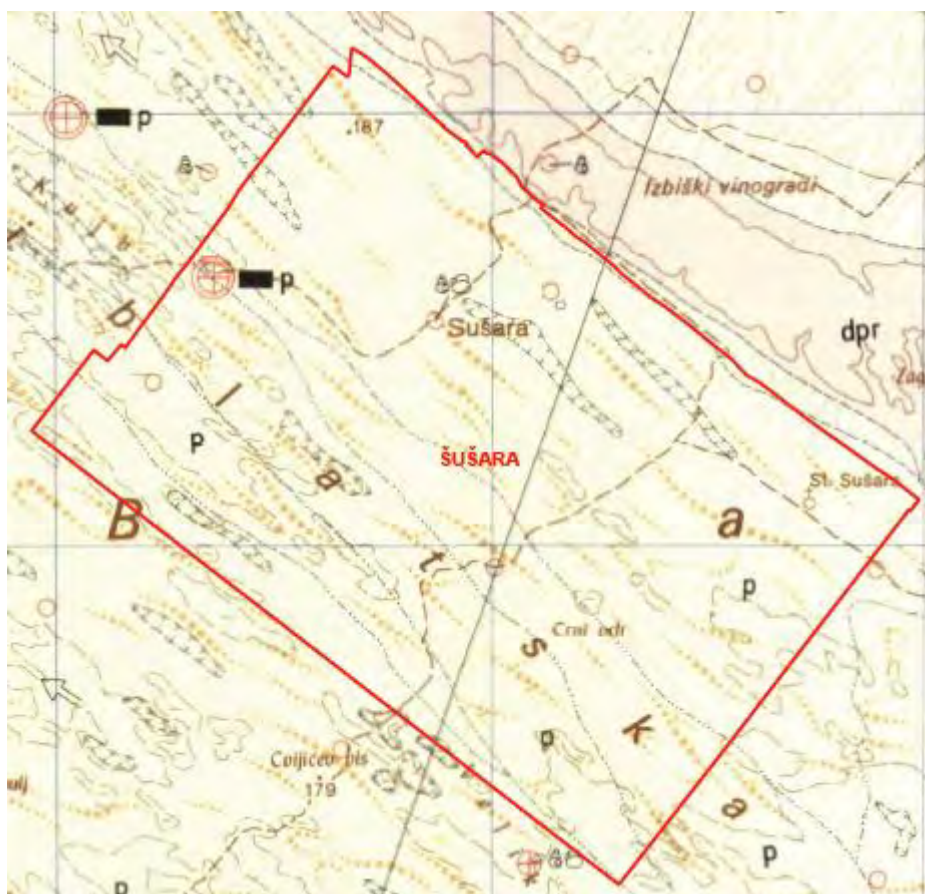
Слика 4: Геолошка карта КО Шушара
