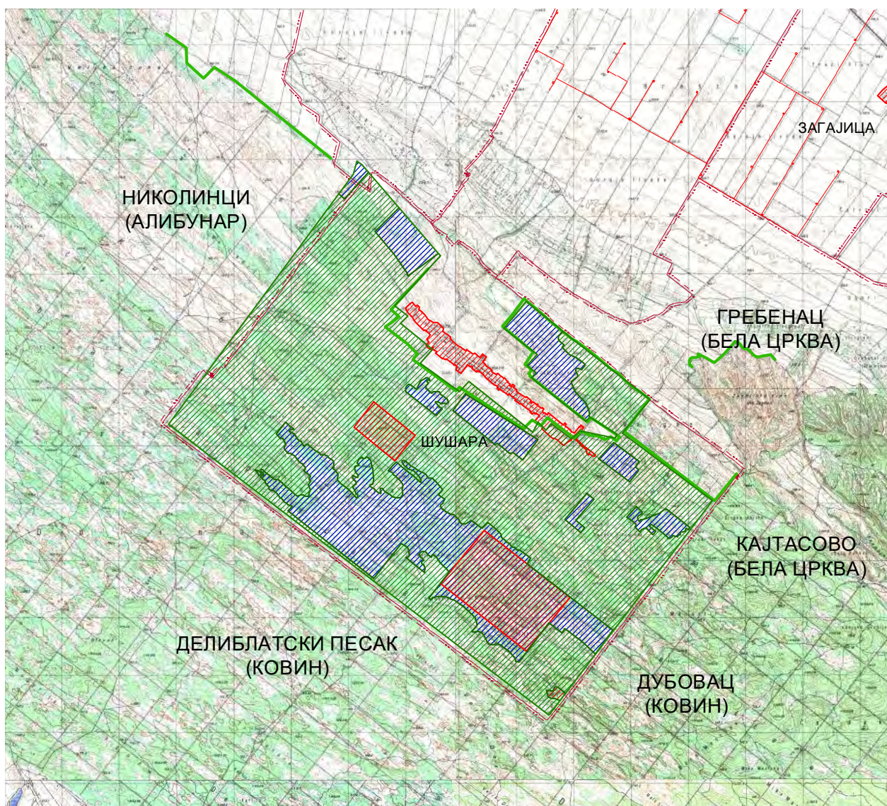
Слика 10: Станишта природних реткости од националног значаја
