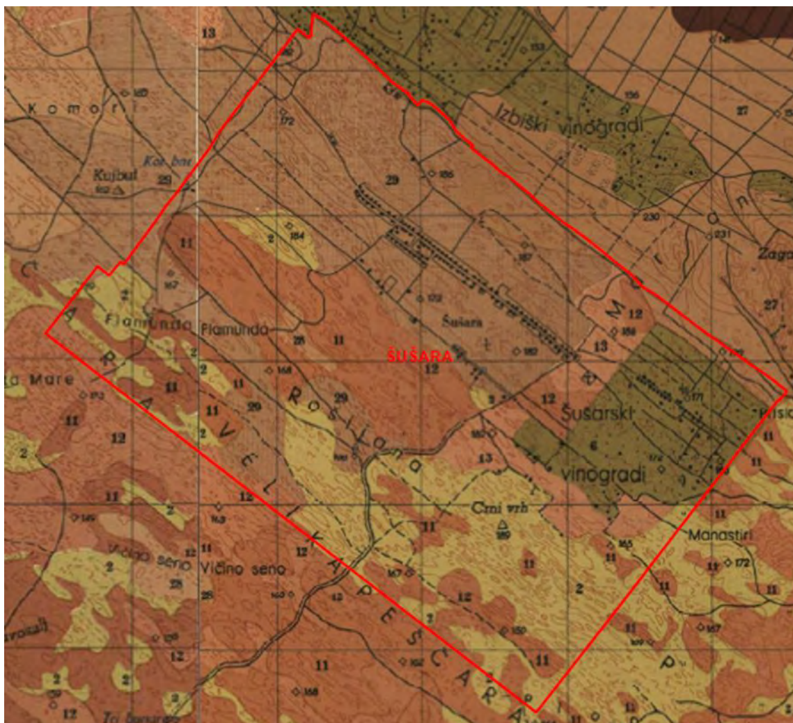
Слика 7: Педолошка карта КО Шушара
