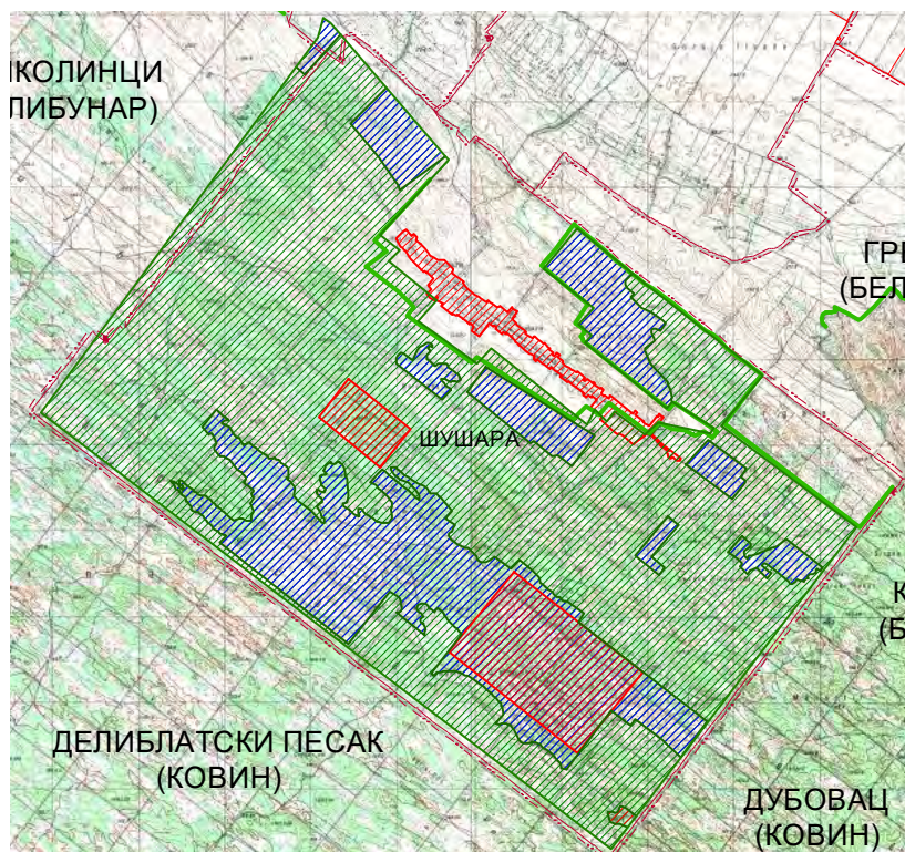
Слика 9: Предлог мрже пољозаштитних појасева у КО Шушара
