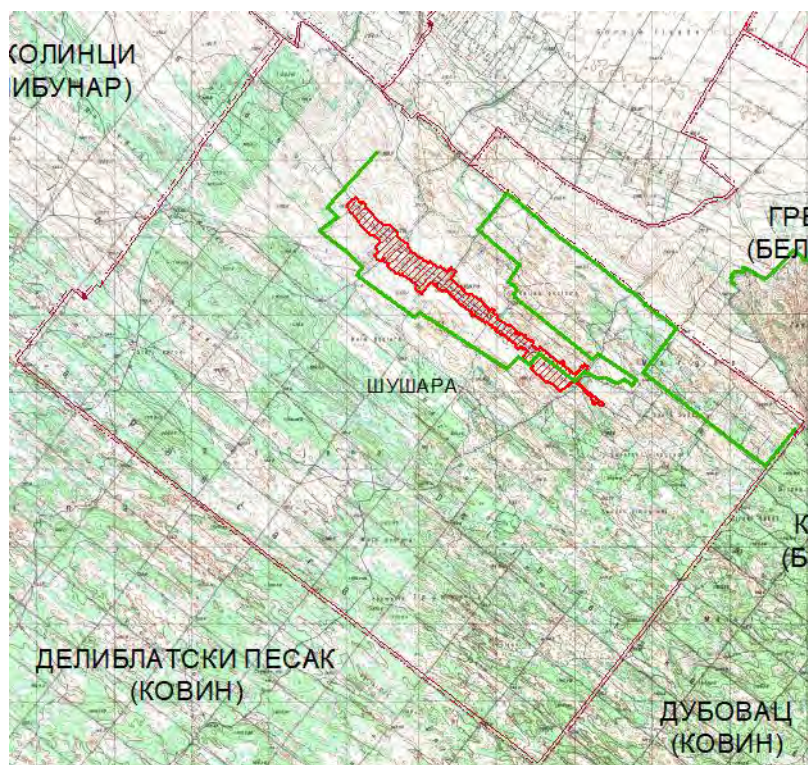
Слика 2: Мрежа водотокова и канала на КО Шушара
